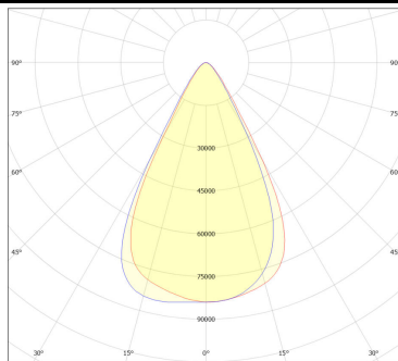
Symmetric optic/symetická optika
