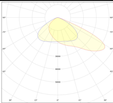
Asymmetric optic/asymetická optika
