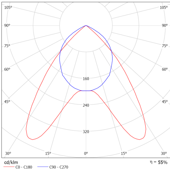
PAR 2X54W
